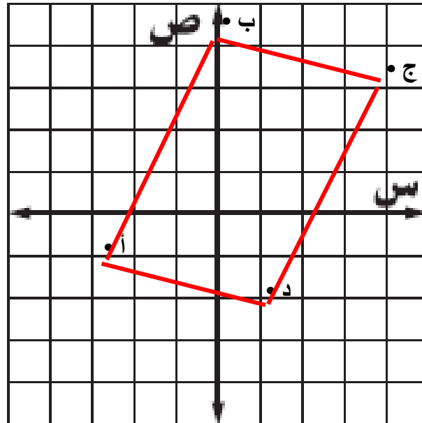
الشكل الناتج متوازي أضلاع أ ب ج د
